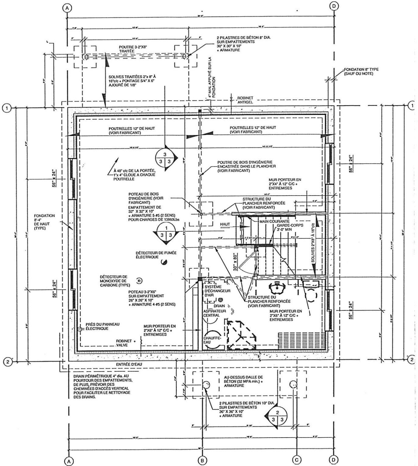
PLAN des FONDATIONS
